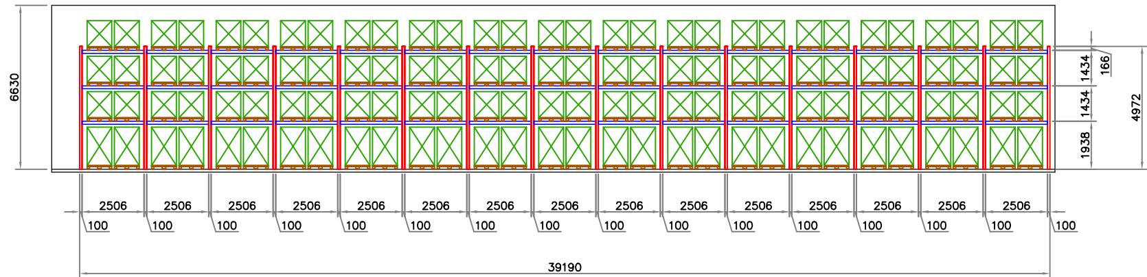
VISTA FRONTALE SCAFFALI FISSI
