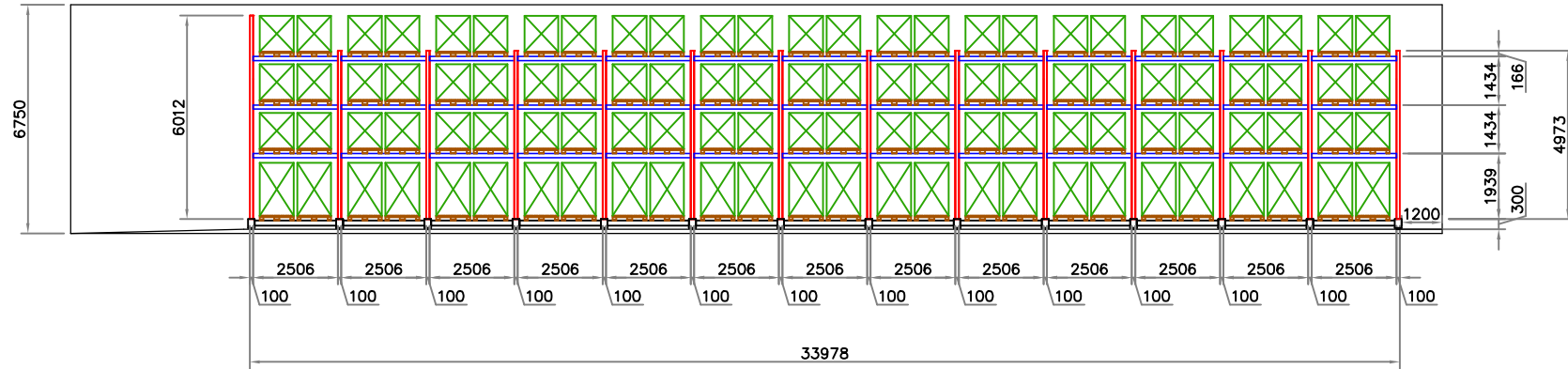
VISTA FRONTALE SCAFFALI FISSI
