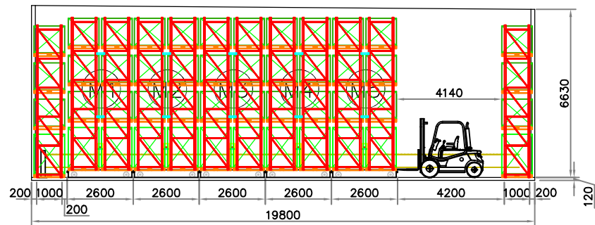
VISTA LATERALE COMPATTABILE
